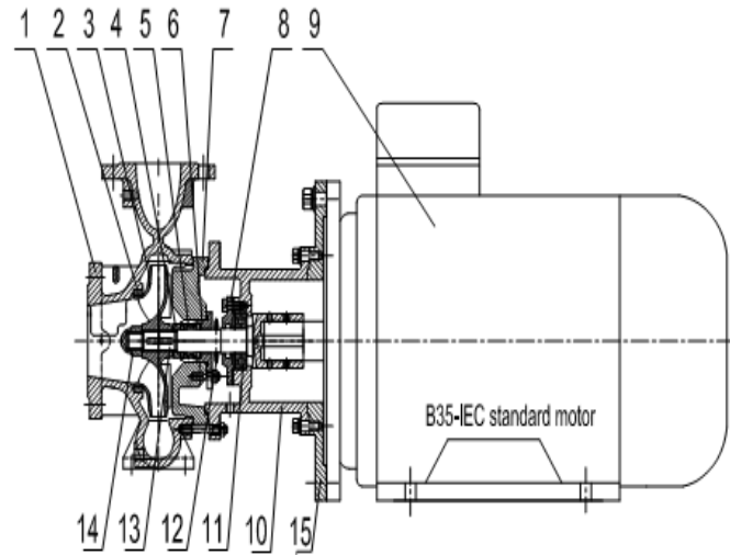
Рисунк1:Агрегат электронасосный NES
